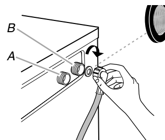
A. Valve du tuyau d'alimentation d'eau froide B. Valve du tuyau d'alimentation d'eau chaude
